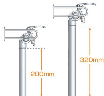
ポスト(サイズ2種類)
