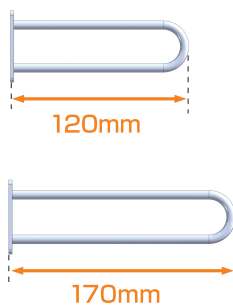
前後調整金物(サイズ2種類)
